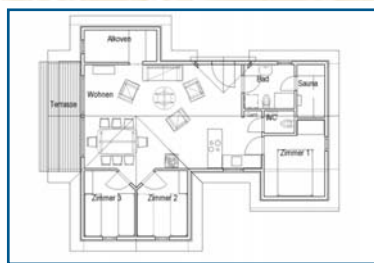
Haustyp E: 6+2 Pers. inkl. Sauna + Alkoven
