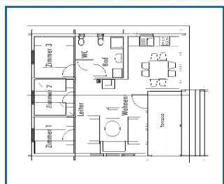
Haustyp D: 6+2 Pers. ohne Sauna + Schlafempore
